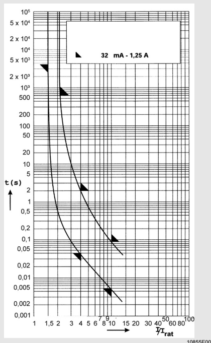
8560/51-...1 250 В среднеинерционный
