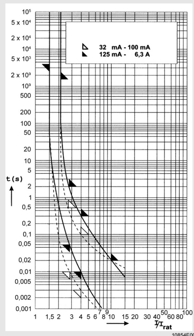
8560/51-...3 250 В безынерционный
