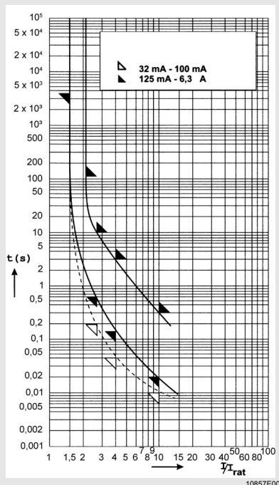
8560/51-...2 250 В инерционный
